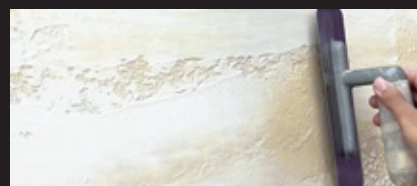
Membuat Motif Marmer Travertine Dalam keadaan basah, tarik cat yang telah diaplikasi secara searah (horizontal) menggunakan roskam stainless steel.
